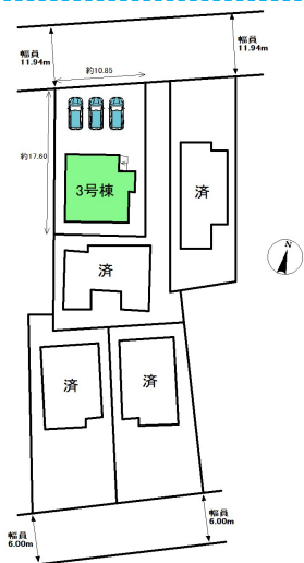
配置図
