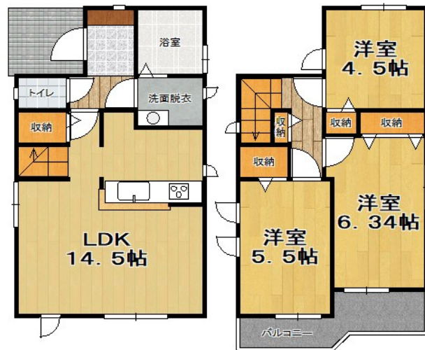
間取図
