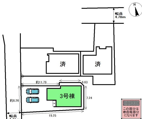
配置図
