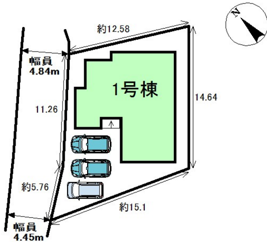
配置図
