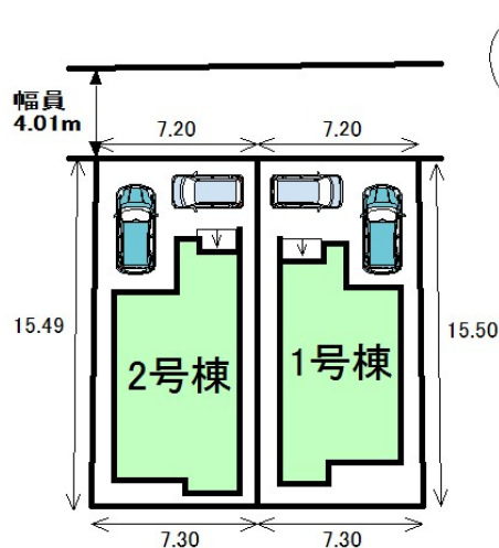
配置図
