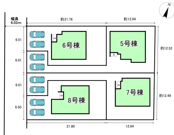
配置図
