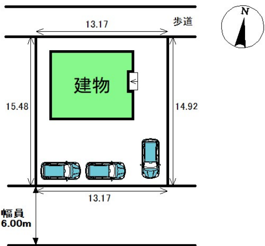
配置図
