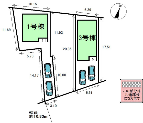
配置図
