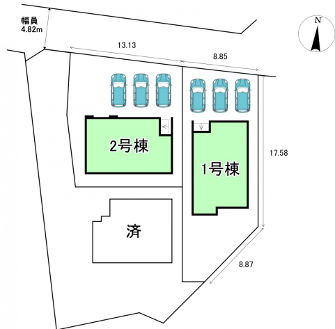
配置図
