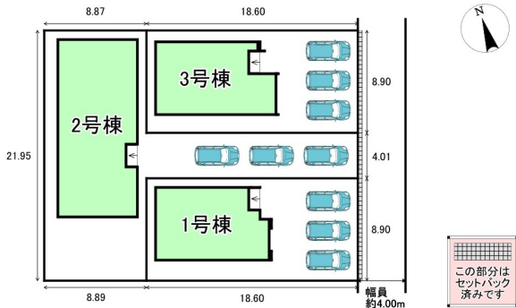
配置図
