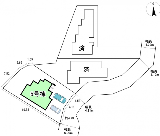
配置図
