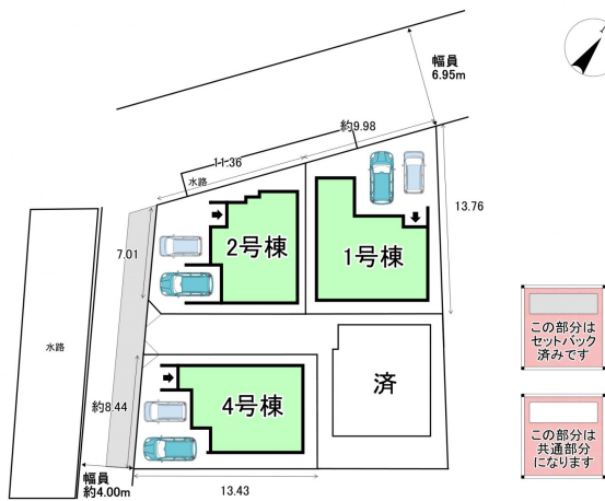
配置図
