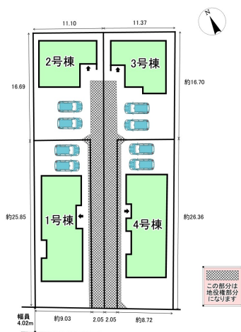
配置図
