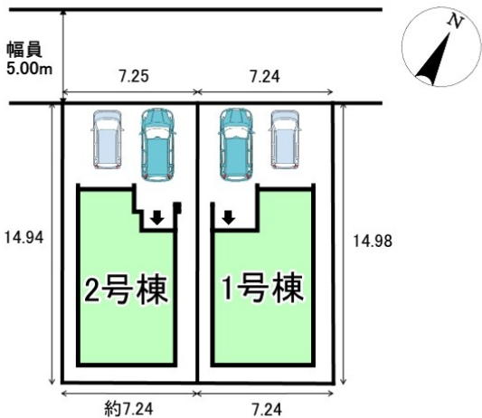
配置図
