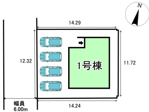
配置図
