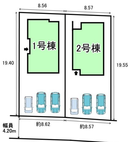
配置図
