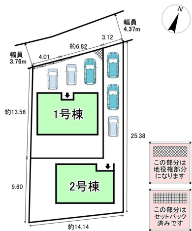
配置図
