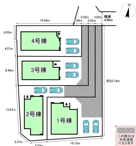
配置図
