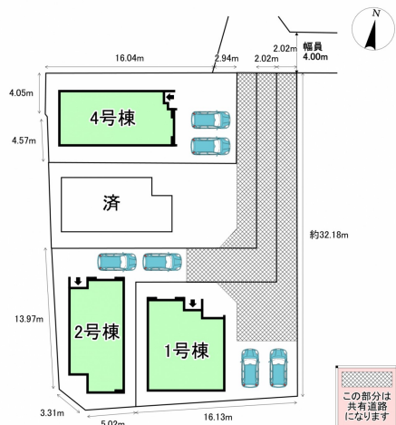
配置図
