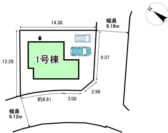
配置図
