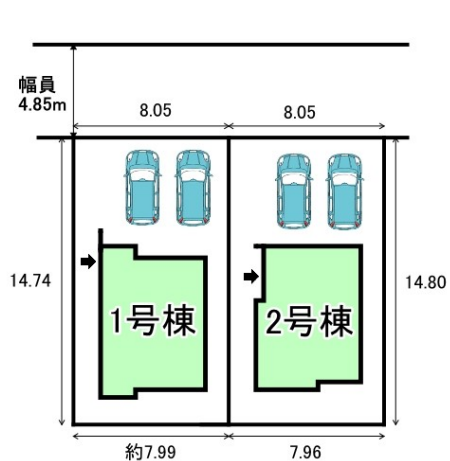
配置図
