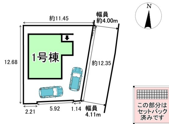
配置図
