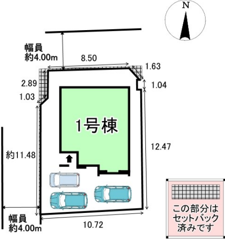
配置図
