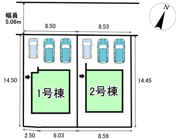
配置図
