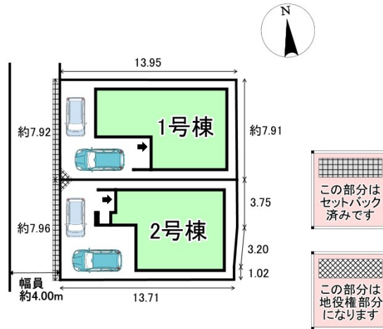
配置図
