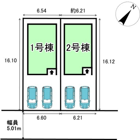
配置図
