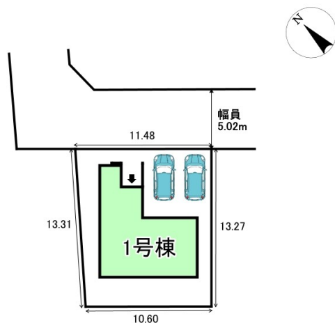
配置図
