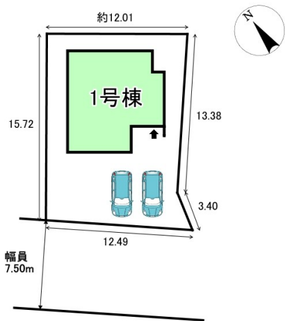
配置図
