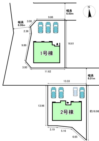
配置図
