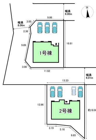
配置図
