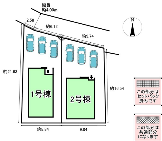
配置図
