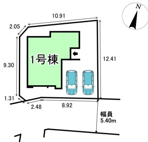
配置図
