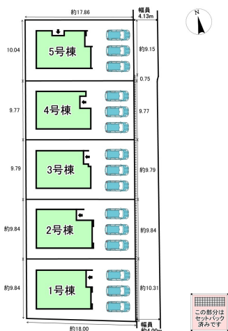
配置図
