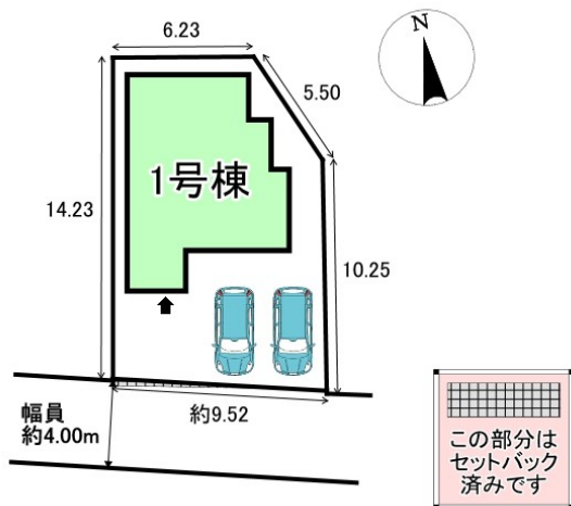
配置図
