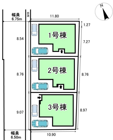
配置図
