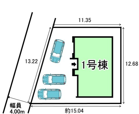
配置図
