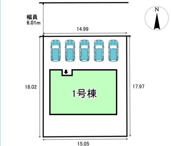
配置図
