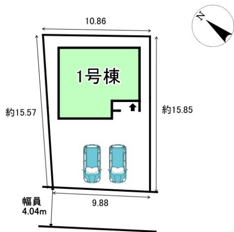
配置図
