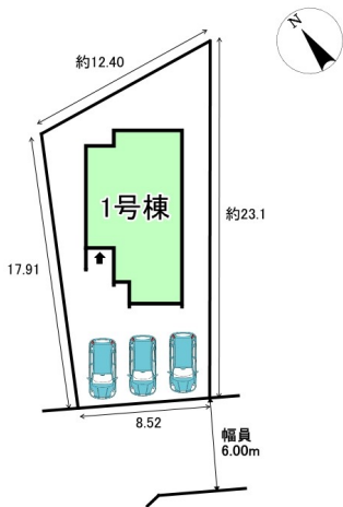
配置図
