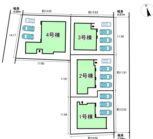
配置図
