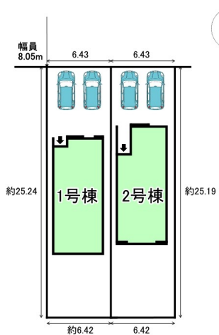
配置図
