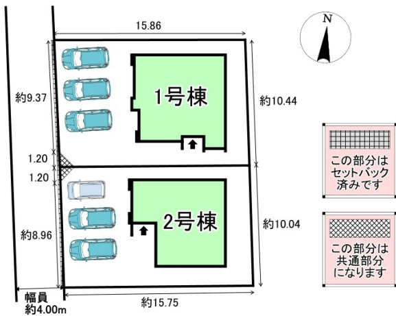
配置図
