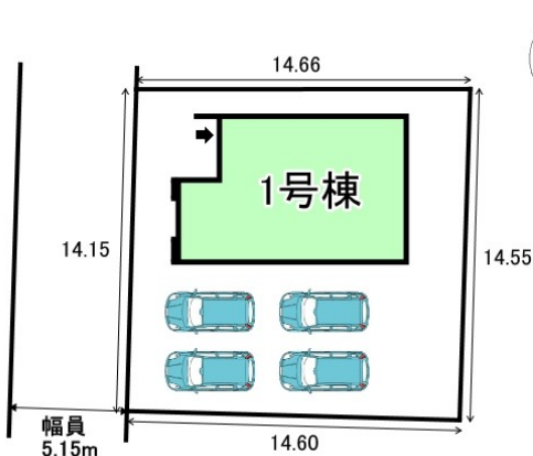
配置図
