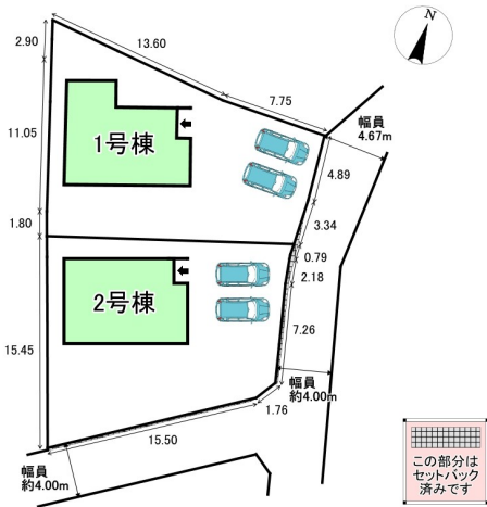
配置図
