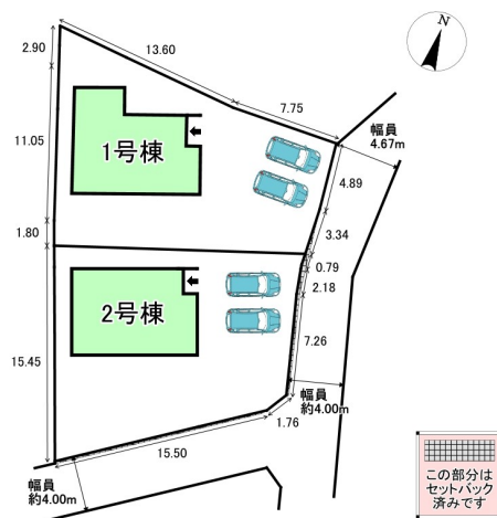
配置図
