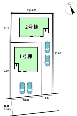
配置図
