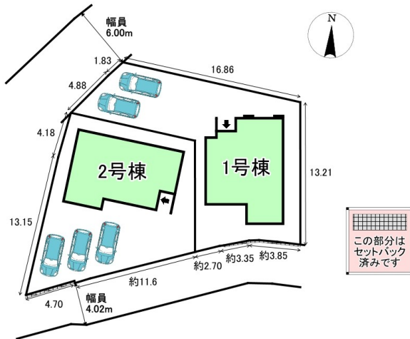
配置図
