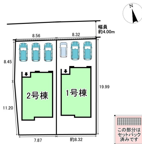
配置図
