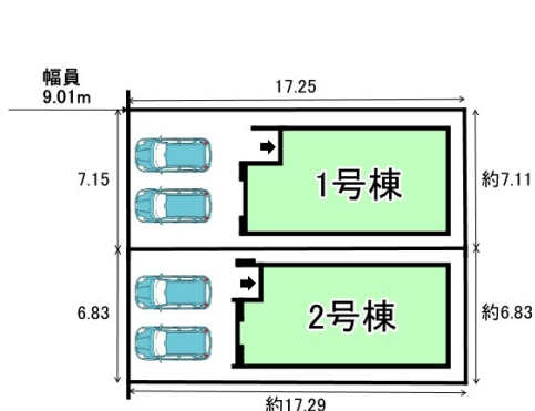
配置図
