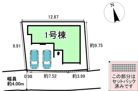
配置図
